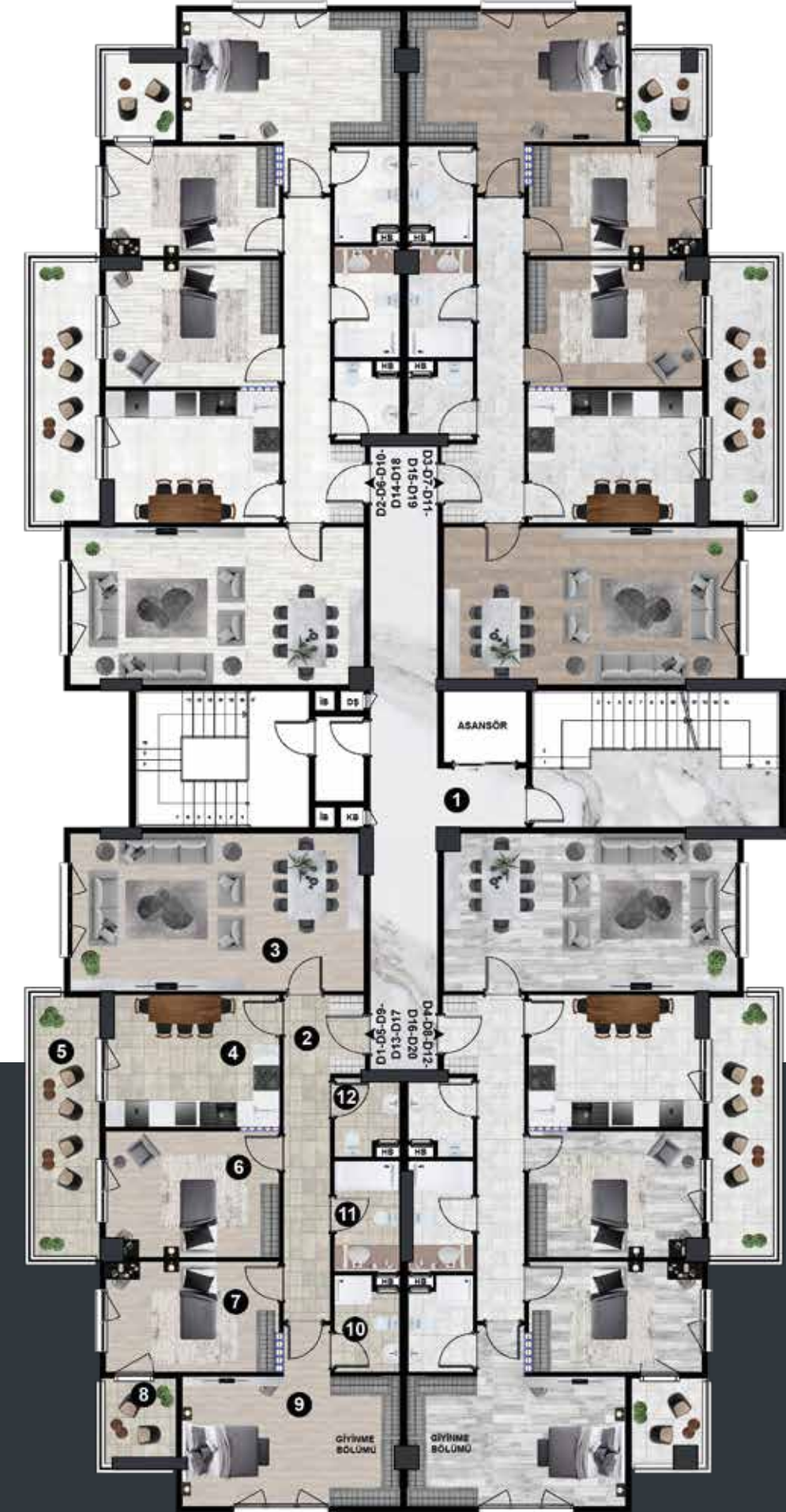
Kat Planı
